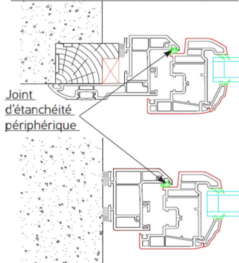
Dormant réno avec aile de 42 mm
