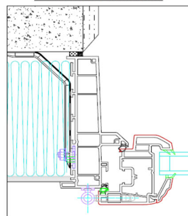
Dormant réno avec aile de 42 mm
